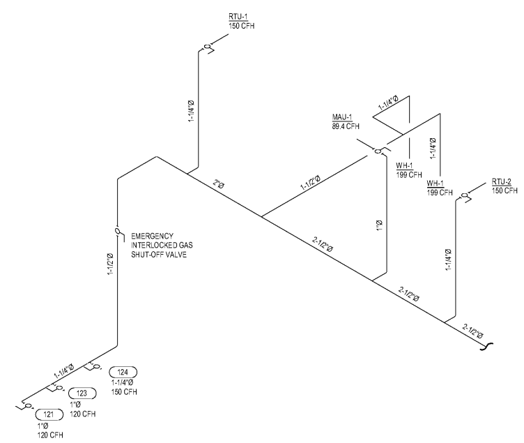
2 GAS RISER DIAGRAMS N.T.S.
