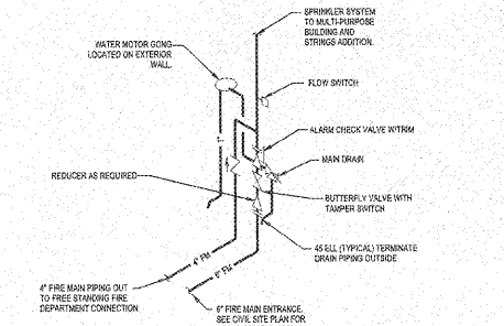
NEW SPRINKLER ENTRANCE RISER SCALE: NONE
