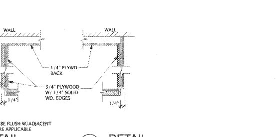
30 DETAIL SCALE: 3\"/>
