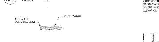
18 SHELF EDGE DETAIL SCALE: 3\"/>
