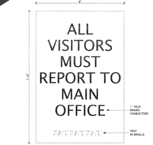
6 SIGN TYPE "E" SCALE: 6" = 1'-0"
