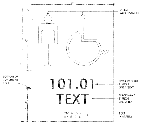
3 SIGN TYPE "B2" SCALE: 6" = 1'-0"
