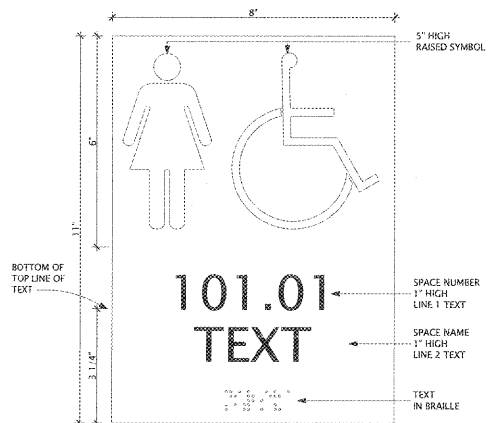
2 SIGN TYPE "B1" SCALE: 6" = 1'-0"
