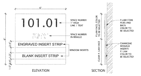
1 SIGN TYPE "A" SCALE: 6" = 1'-0"
