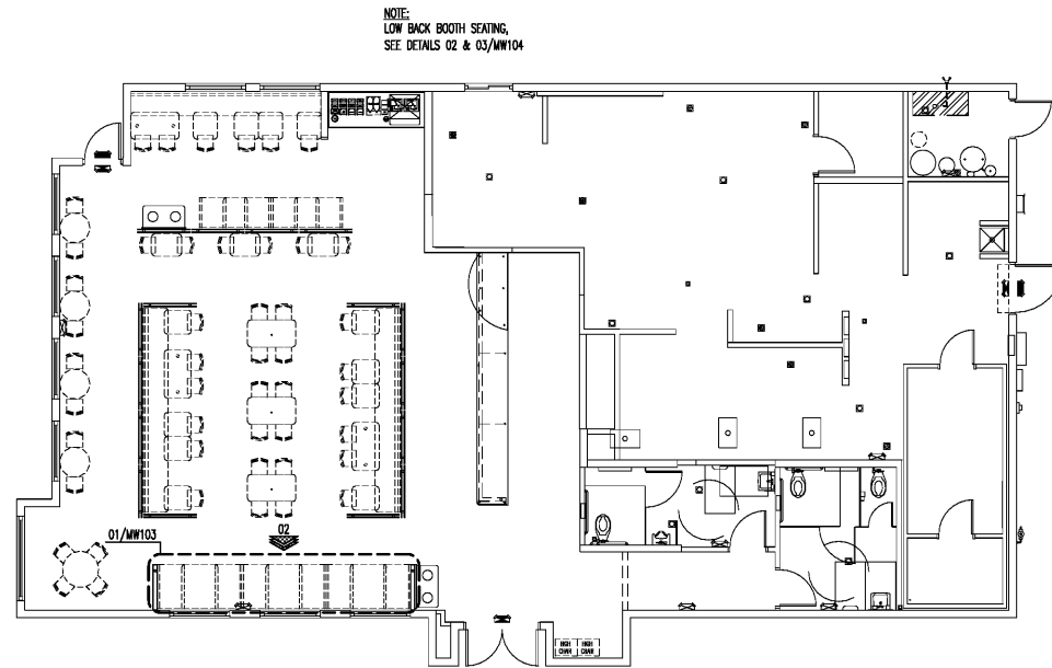
05 KEY PLAN SCALE: 1/8"=1'-0"
