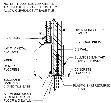
2 TILE BASE AT DIE WALL Scale: 3" = 1'-0"
