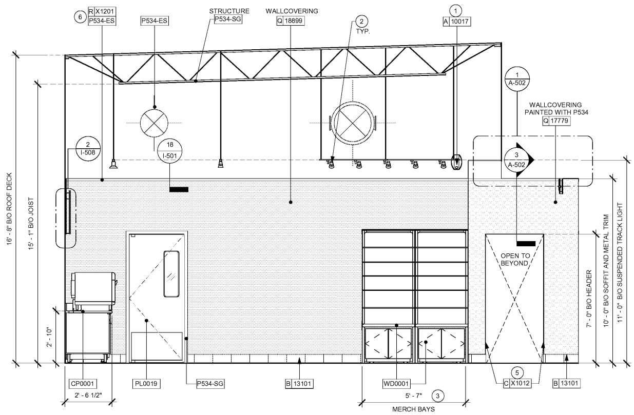
1 MERCH BAYS Scale: 3/8" = 1'-0"
