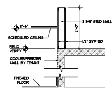
(D) PONY WALL DETAIL SCALE: 3/4" = 1'-0"
