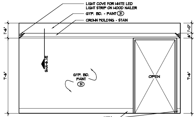
A INTERIOR ELEVATION SCALE: 3/8" = 1'-0"
