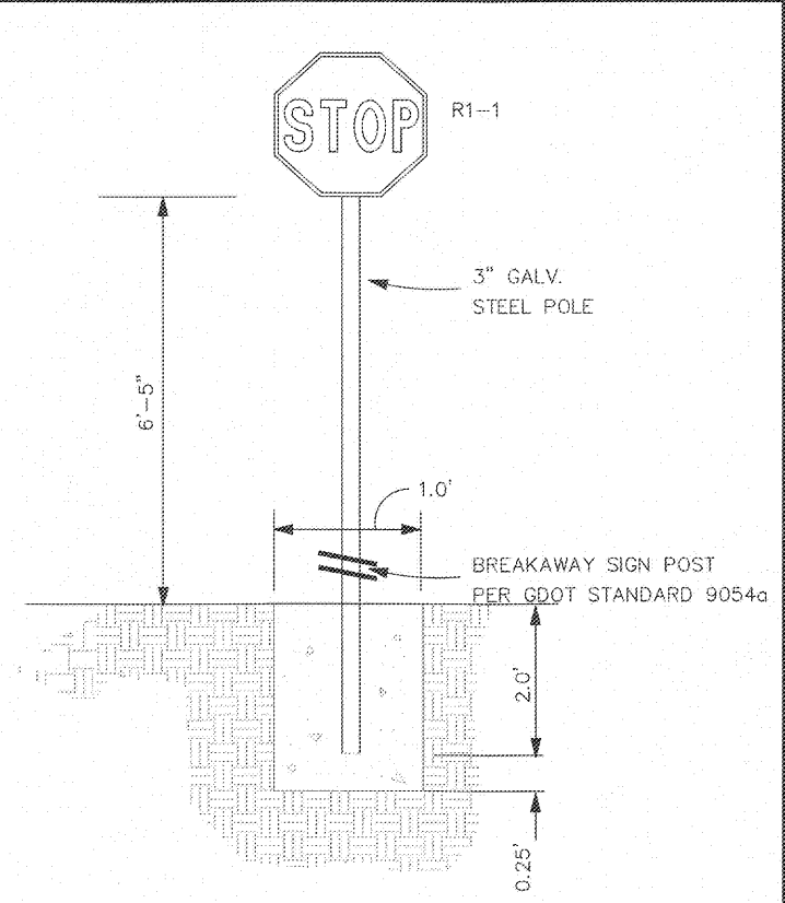
STOP SIGN N.T.S. CS44
