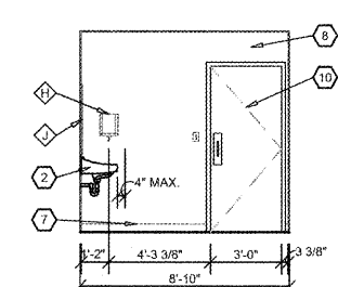
8 ELEVATION A4.1 SCALE: 1/4" = 1'-0"
