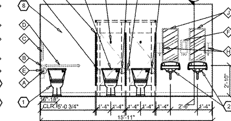
7 ELEVATION A4.1 SCALE: 1/4" = 1'-0"
