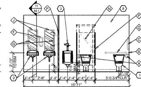
3 ELEVATION A4.1 SCALE: 1/4" = 1'-0"
