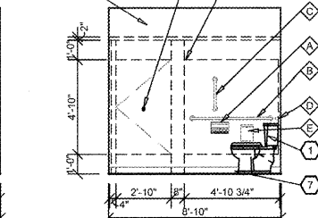
6 ELEVATION A4.1 SCALE: 1/4" = 1'-0"
