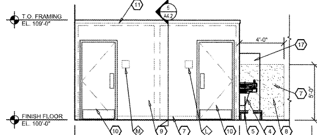
13 ELEVATION A4.1 SCALE: 1/4" = 1'-0"
