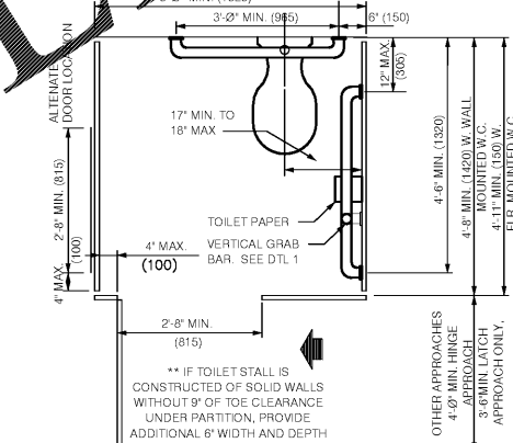
STANDARD TOILET STALL N.T.S. 2
