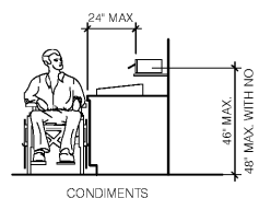
REACH RANGES N.T.S. 14
