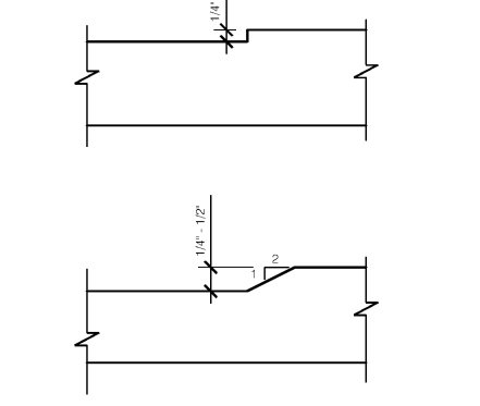
CHANGES IN LEVEL N.T.S. 12
