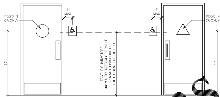
ACCESSIBLE RESTROOM DOORS N.T.S. 15
