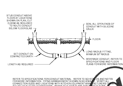
20 BEVERAGE CONDUIT BELOW SLAB NTS
