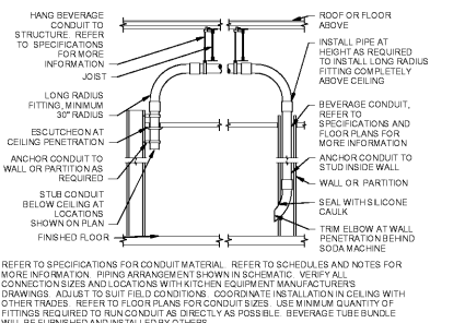
19 ABOVE-CEILING BEVERAGE CONDUIT NTS
