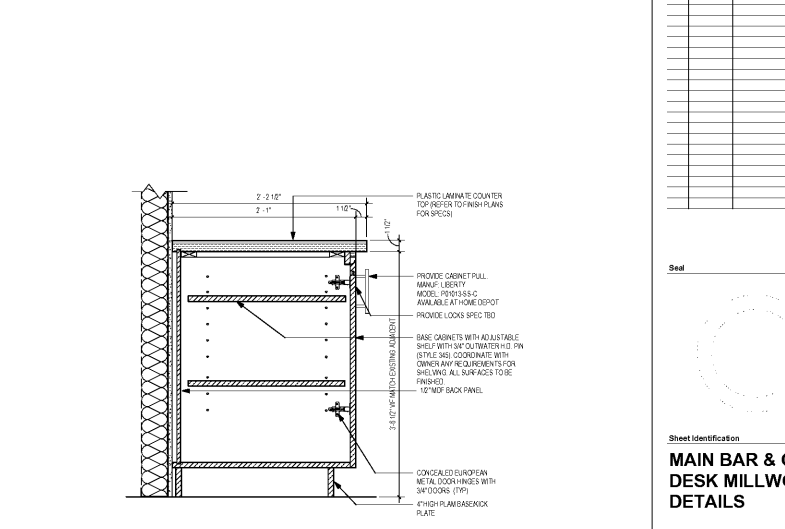
A3 BACK BAR CABINET 1/8" = 1'-0"
