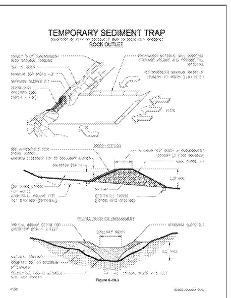
9 TEMPORARY SEDIMENT TRAP SCALE: 1/4" = 1'-0"
