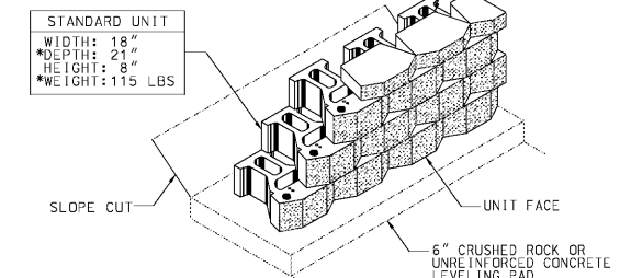
1 STANDARD UNIT/BASE PAD ISOMETRIC VIEW SCALE: 3/8" = 1'-0"
