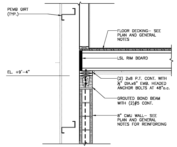
SECTION 2 SCALE: 3/4" = 1'-0" S3-4
