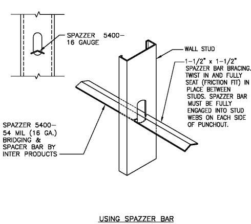
USING SPAZZER BAR
