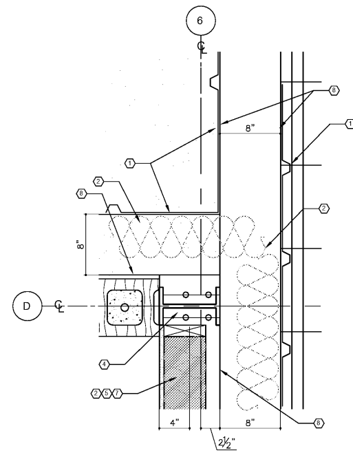
2 COLUMN DETAIL AS-3 SCALE: 1-1/2" = 1'-0"
