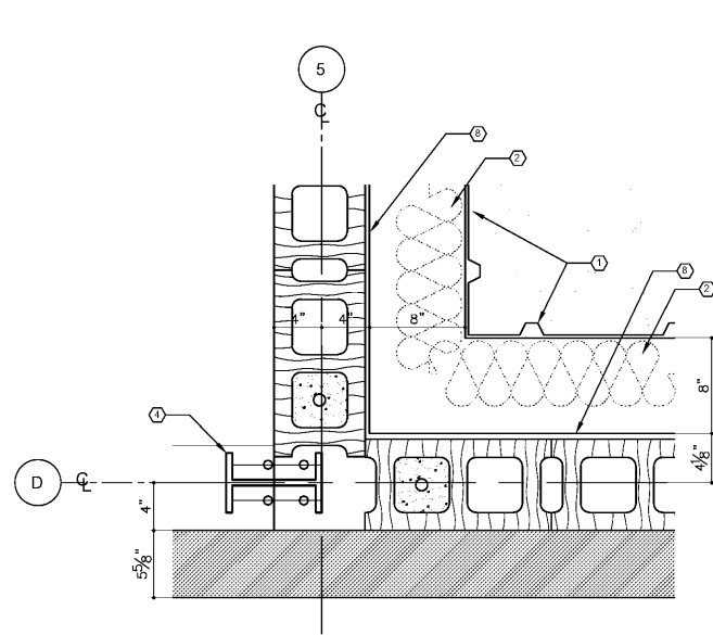
1 COLUMN DETAIL AS-3 SCALE: 1-1/2" = 1'-0"
