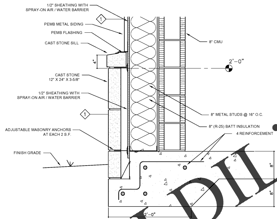
3 A2-9 ADD. ALT. NO.1 SCALE: 1-1/2" = 1'-0"
