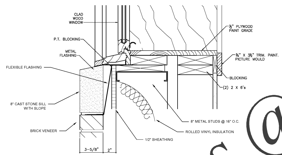
2 A2-9 SILL - WINDOW SCALE: 3" = 1'-0" ADD. ALT. NO.2
