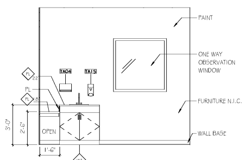
A4 CLS PATIENT RM 214 - E SCALE: 3/8" = 1'-0"
