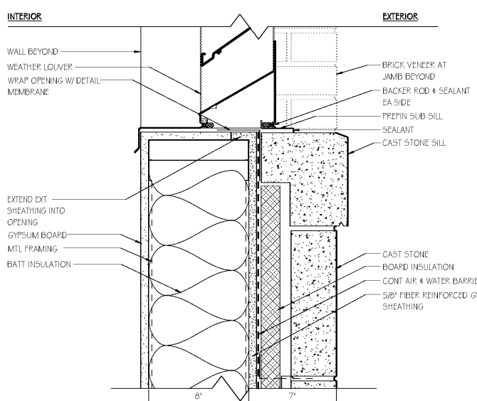
A10 LOUVER SILL SCALE: 3" = 1'-0"
