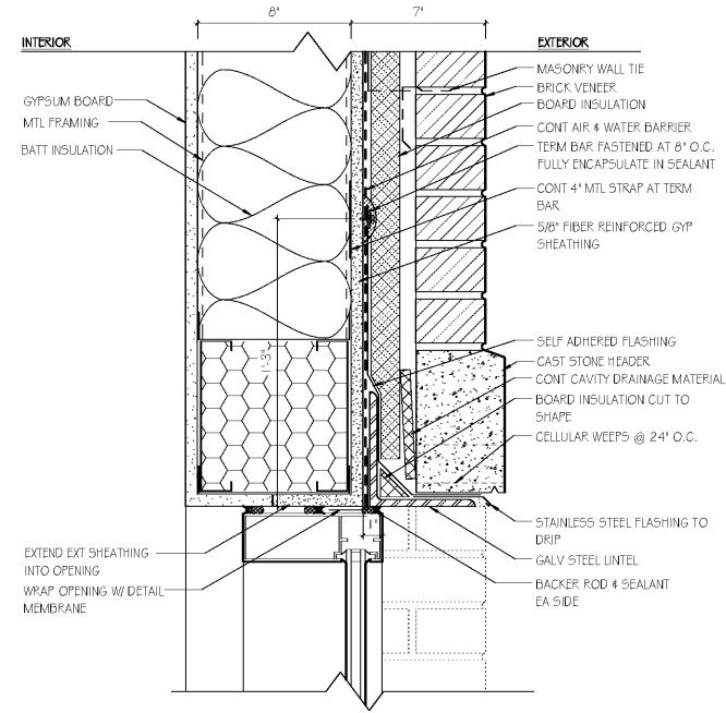
G6 EXT GYP - CW HEAD SCALE: 3" = 1'-0"
