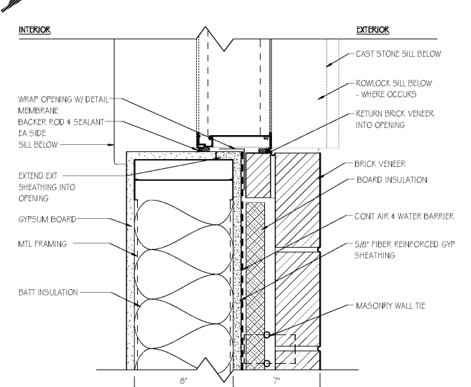
D10 LOUVER JAMB SCALE: 3" = 1'-0"
