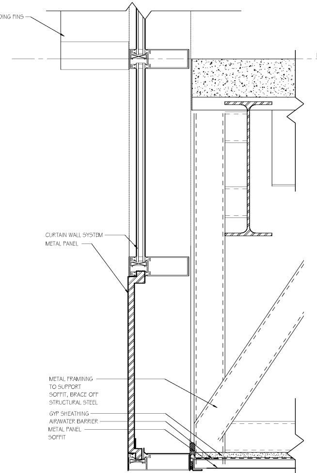
A9 CANTILEVER FLOOR SCALE: 3" = 1'-0"
