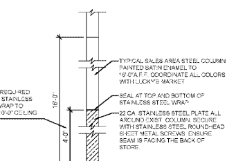
13 COLUMN WRAP DETAIL SCALE: 1/2" = 1'-0"
