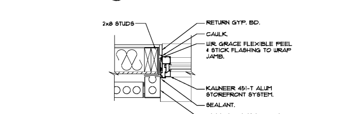
7 JAMB DETAIL 1 1/2" x 1'-0"
