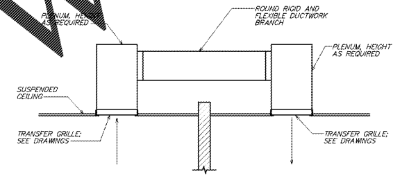
8 RETURN AIR TRANSFER SCALE: NONE
