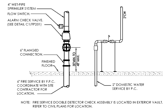
A1 Fire Protection Riser Detail SCALE: N.T.S.
