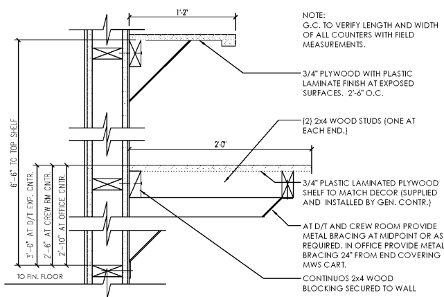
07 COUNTER SECTION A7.1 SCALE: 3/8" = 1'-0"
