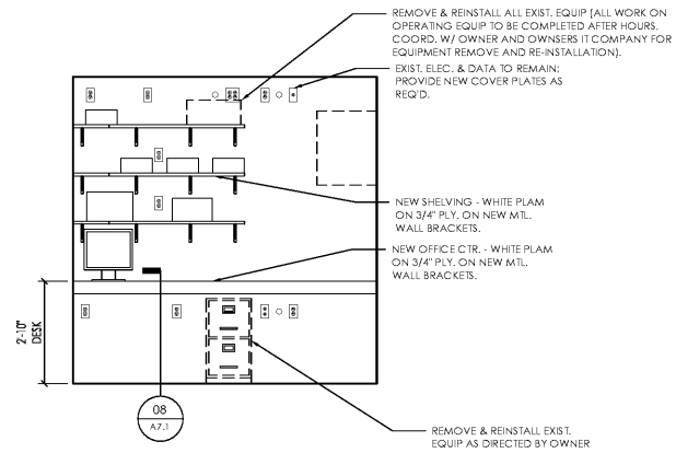
08 OFFICE A7.1 SCALE: 3/8" = 1'-0"
