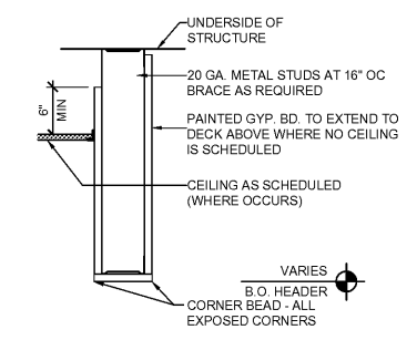
2 SOFFIT SECTION SCALE: N.T.S.
