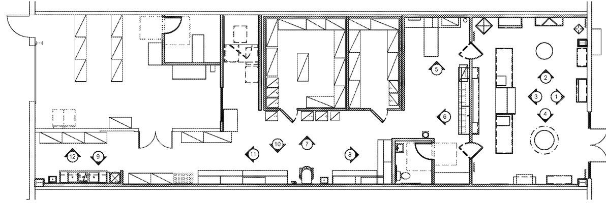
A KEY PLAN SCALE: 1/8" = 1'-0"
