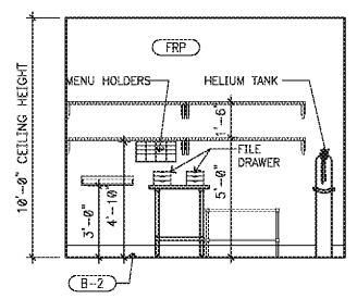
5 INT. ELEVATION SCALE: 1/4" = 1'-0"
