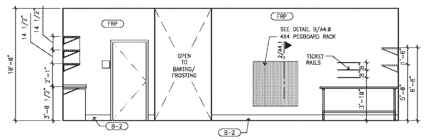
6 INT. ELEVATION SCALE: 1/4" = 1'-0"
