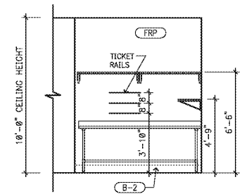
8 INT. ELEVATION SCALE: 1/4" = 1'-0"
