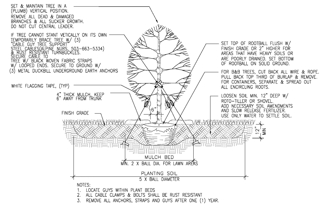
B1 TREE DETAIL N.T.S.
