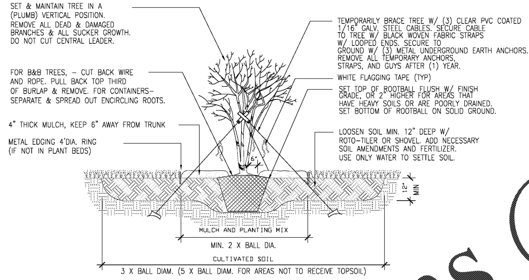
D1 MULTI-STEMMED TREE DETAIL N.T.S.
