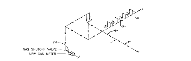
3 GAS RISER DIAGRAM P2.1 N.T.S.
