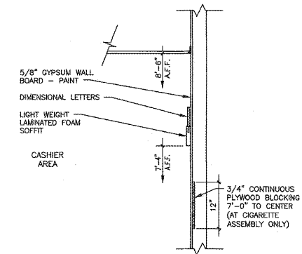
2 SOFFIT DETAIL • CHECKOUT A3.1 SCALE: 3/4" = 1'-0"
