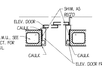
5 JAMB DETAIL SCALE: 1" = 1'-0"
