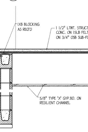
6 HEAD & SILL DETAIL SCALE: 1" = 1'-0"
