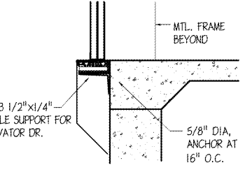
4 SILL DETAIL SCALE: 1" = 1'-0"
