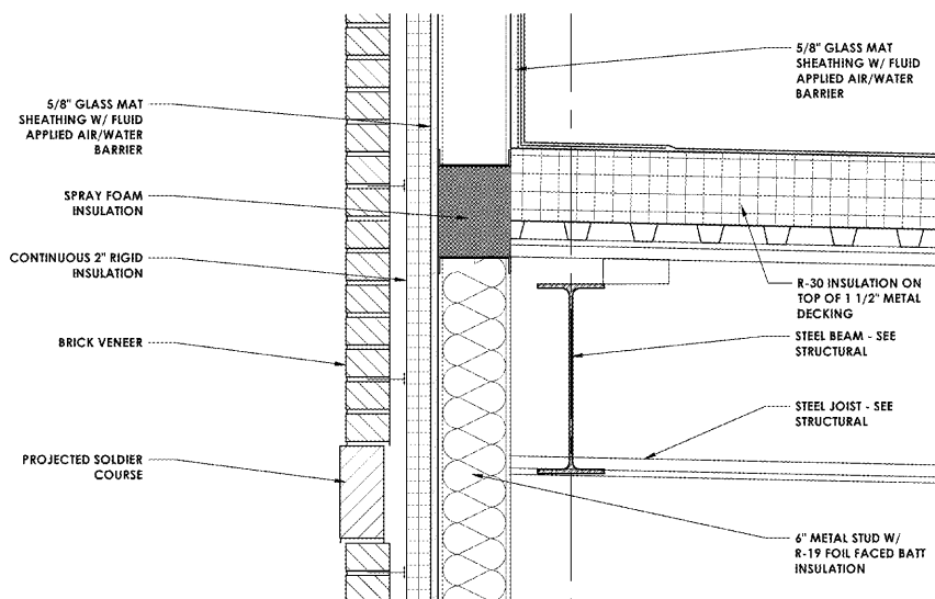
8 DETAIL SECTION Scale: 1-1/2" = 1'-0"
