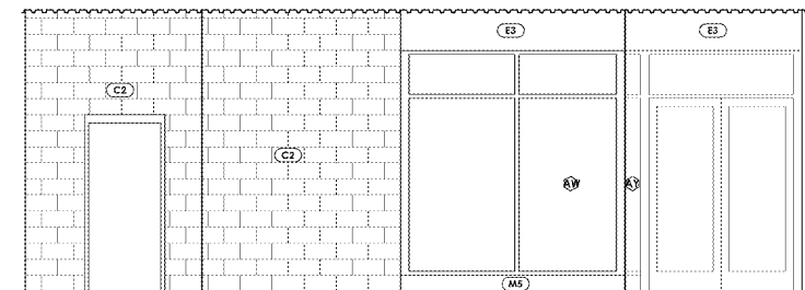
2 ELEVATION Scale: 1/4" = 1'-0"
