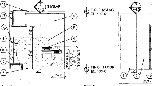
12 ELEVATION A4.1 SCALE: 1/4" = 1'-0"
