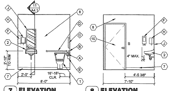
7 ELEVATION A4.1 SCALE: 1/4" = 1'-0"
