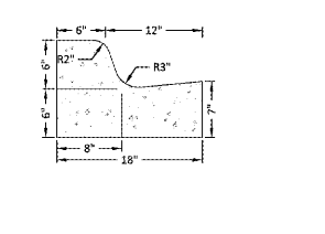
WAWA TYPE F1 CURB NTS
