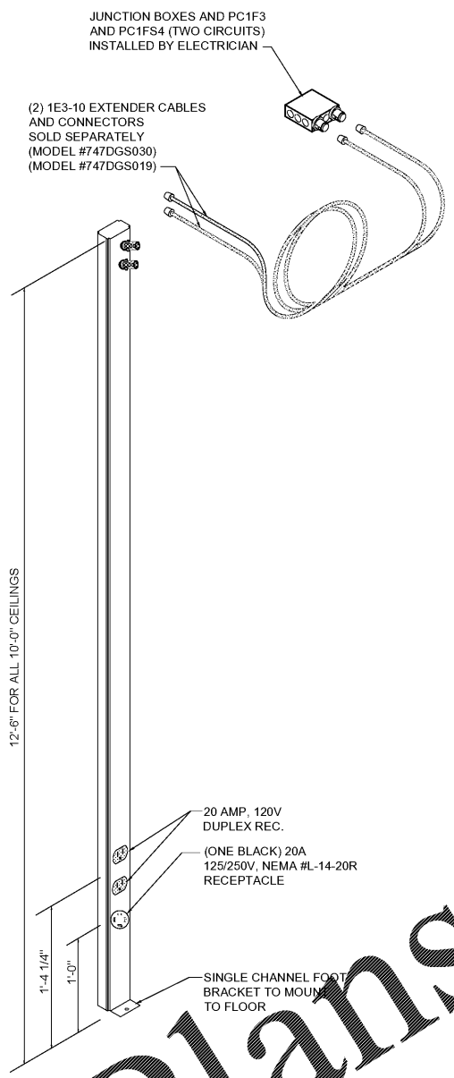
747DGS020-12BK COOLER/FREEZER POWER POLE Scale: N.T.S.
