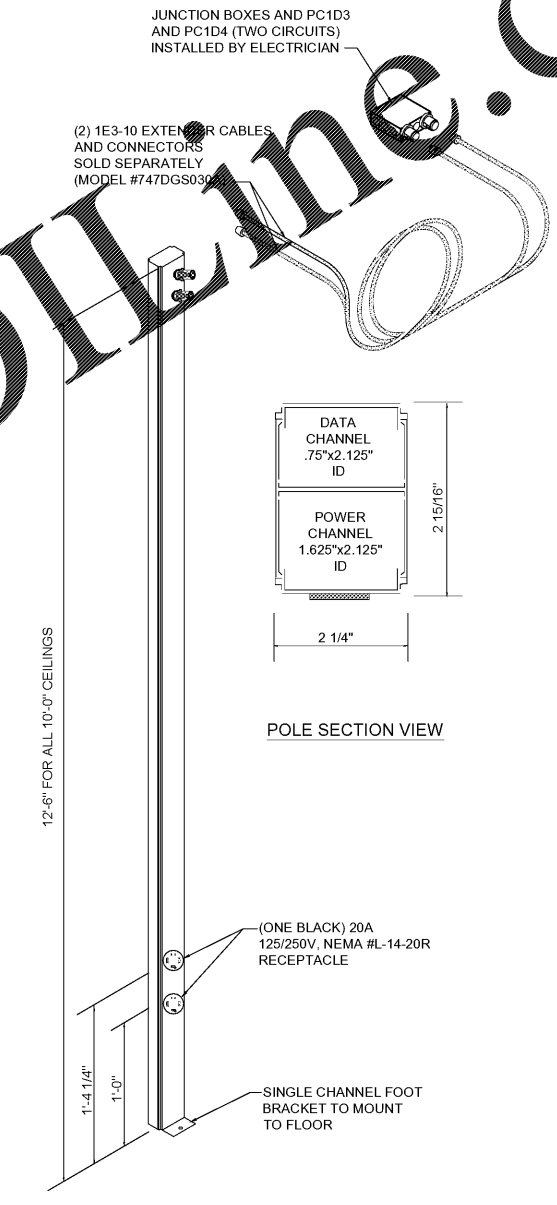
747DGS030-12' FREEZER POWER POLES Scale: N.T.S.
