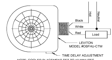
2 "B" OCCUPANCY SENSOR N.T.S.
