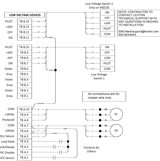
7 IRC WIRING DIAGRAM N.T.S.
