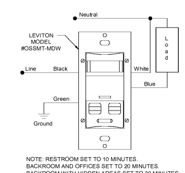
1 "A" OCCUPANCY SENSOR N.T.S.
