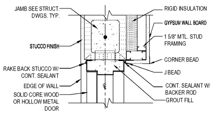
06 JAMB DETAIL SCALE: 1/12"=1'-0"
