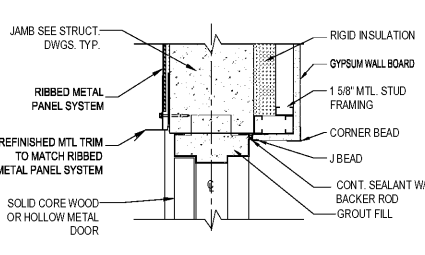
08 JAMB DETAIL SCALE: 1/12"=1'-0"
