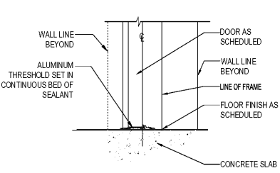
11 SILL DETAIL SCALE: 1/12"=1'-0"
