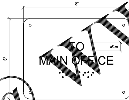
D3 SIGN TYPE SCALE: 6"=1'-0"
