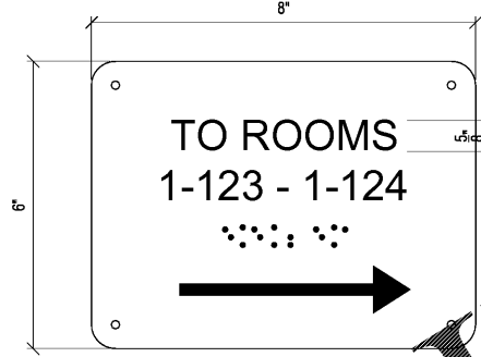
D1 SIGN TYPE SCALE: 6"=1'-0"
