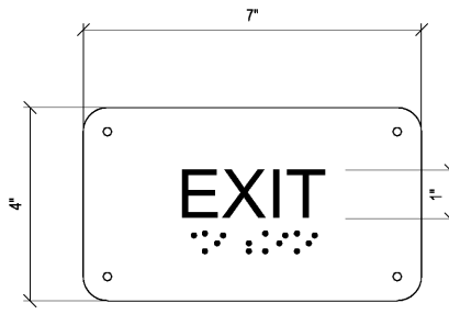
F SIGN TYPE SCALE: 6"=1'-0"
