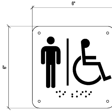
E1 SIGN TYPE SCALE: 6"=1'-0"
