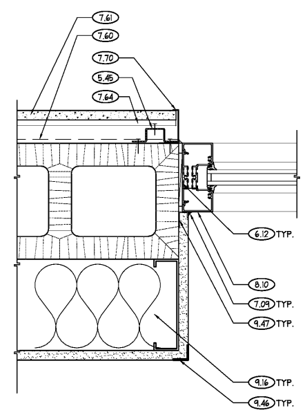
1 PLAN DETAIL SCALE: 3" = 1'-0"
