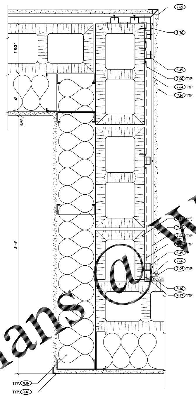
2 PLAN DETAIL SCALE: 3" = 1'-0"
