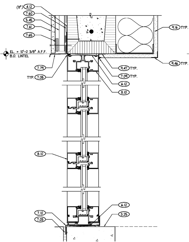
2 STOREFRONT HEAD/ SILL DETAIL SCALE: 3" = 1'-0"
