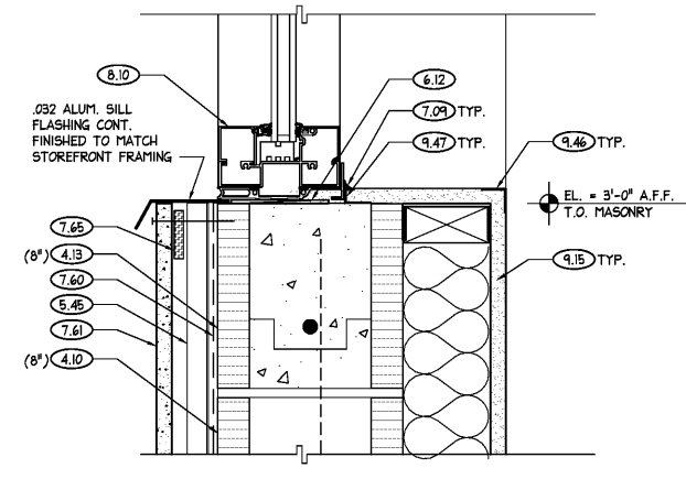
10 SILL DETAIL SCALE: 3" = 1'-0"
