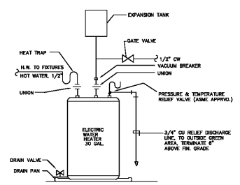
3 WATER HEATER DETAIL P1 SCALE: N.T.S.
