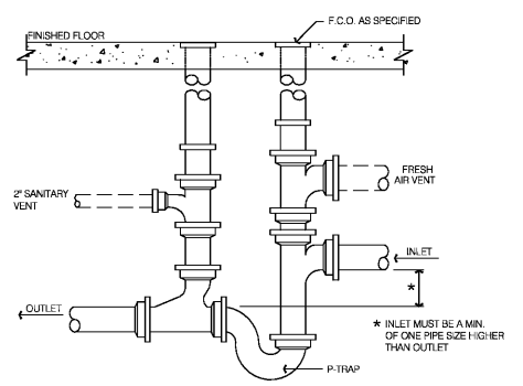
2 MASTER TRAP DETAIL P1 SCALE: N.T.S.
