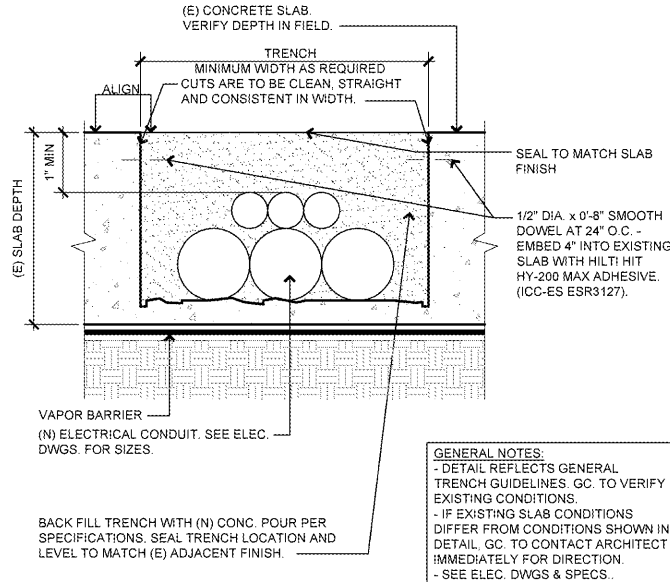
SECTION THRU TRENCH SCALE: 6\"/>
