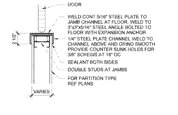
20 JAMB 1 1/2" x 1'-0"
