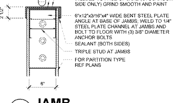
16 JAMB 1 1/2" x 1'-0"
