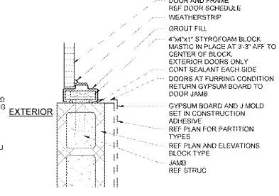
14 JAMB 1 1/2" x 1'-0"
