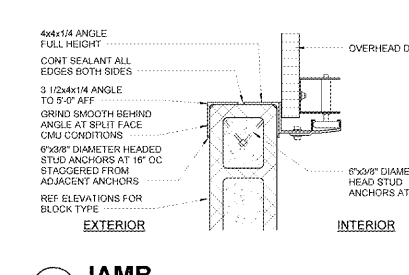
7A JAMB 1 1/2" x 1'-0"
