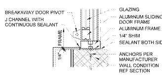
4A JAMB 1 1/2" x 1'-0"
