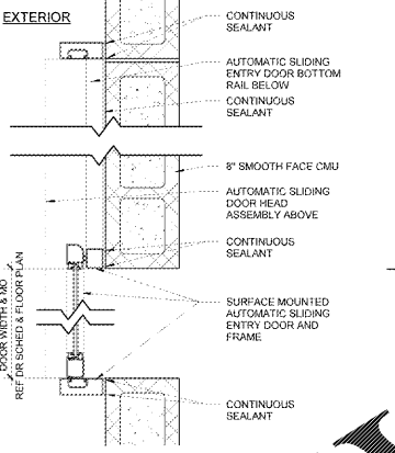
19A JAMB 1 1/2" x 1'-0"
