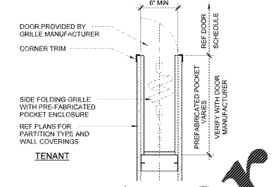
27 JAMB 1 1/2" x 1'-0"
