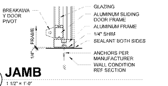
4 JAMB 1 1/2" x 1'-0"
