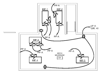
MEZZANINE POWER PLAN SCALE: 1/8" = 1'-0"
