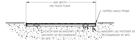
J8 ENTRY FLOOR MAT - SECT 2 SCALE: 3"=1'-0"
