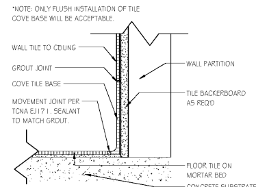
G3 HFT TO HWT SCALE: 3"=1'-0"
