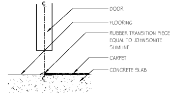
J5 SC TO CPT - TYP SCALE: 3"=1'-0"
