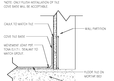
G5 HFT TO HTB DETAIL SCALE: 3"=1'-0"
