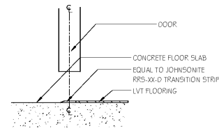
J1 SC TO LVT SCALE: 3"=1'-0"
