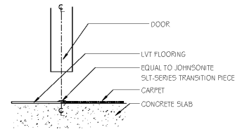
J3 LVT TO CPT SCALE: 3"=1'-0"
