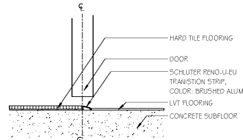
G1 HFT TO LVT SCALE: 3"=1'-0"
