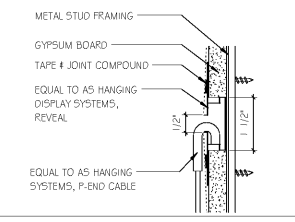
A5 PICTURE HANGING REVEAL SCALE: 6" = 1'-0"
