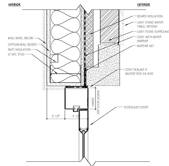
A10 REAR/AUX ENTRY DR JAMB SCALE: 3" = 1'-0"
